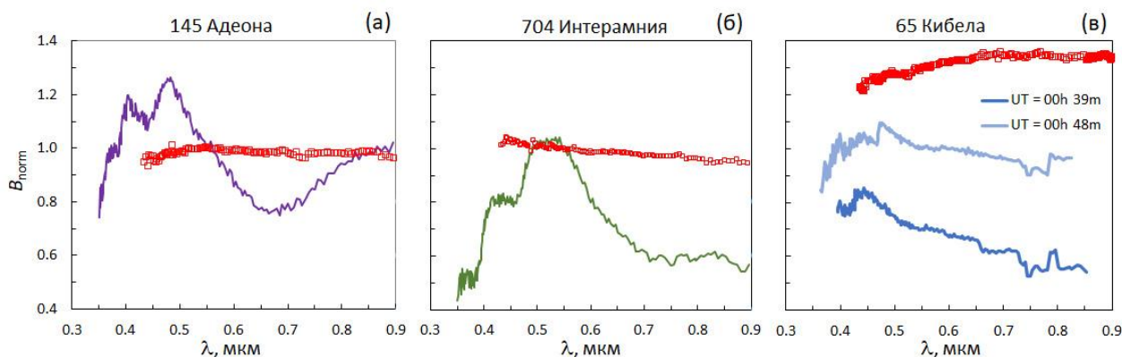
Рис. 1. Спектры отражательной способности V_{\text{norm}} , нормированной на длину волны \lambda = 0.55 мкм, измеренные у астероидов 145 Адеона и 704 Интерамния в сентябре 2012 г. и астероида 65 Кибела в сентябре 2016 г. (Бусарев и др., 2019; и ссылки там). Спектры SMASSII этих астероидов показаны красным. Спектры на панели (в) сдвинуты по вертикали на 0.3 друг относительно друга.
