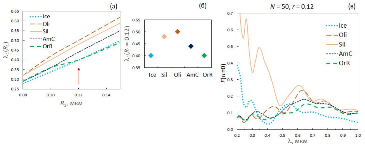
Рис. 8. (а) – Положение первого интерференционного минимума \lambda_1 в спектре для одиночных сферических частиц разного состава в зависимости от радиуса этих частиц R_1 . (б) – Положение \lambda_1 в спектре в зависимости от состава частиц при их радиусе R_1 = 0.12 мкм (отмечено стрелкой на панели (а)). (в) – Спектральные зависимости F(\alpha=0^\circ) для агрегатных частиц разного состава при радиусе мономеров r = 0.12 мкм (структура С).
