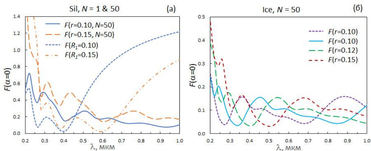
Рис. 5. Спектральные зависимости F(\alpha=0^\circ) для агрегатных (с мономерами указанных радиусов r ) и одиночных частиц (указанных радиусов R_1 ) астрономических силикатов (а) и ледяных агрегатных частиц с мономерами разных размеров (б). Агрегаты типа С содержат 50 мономеров.
