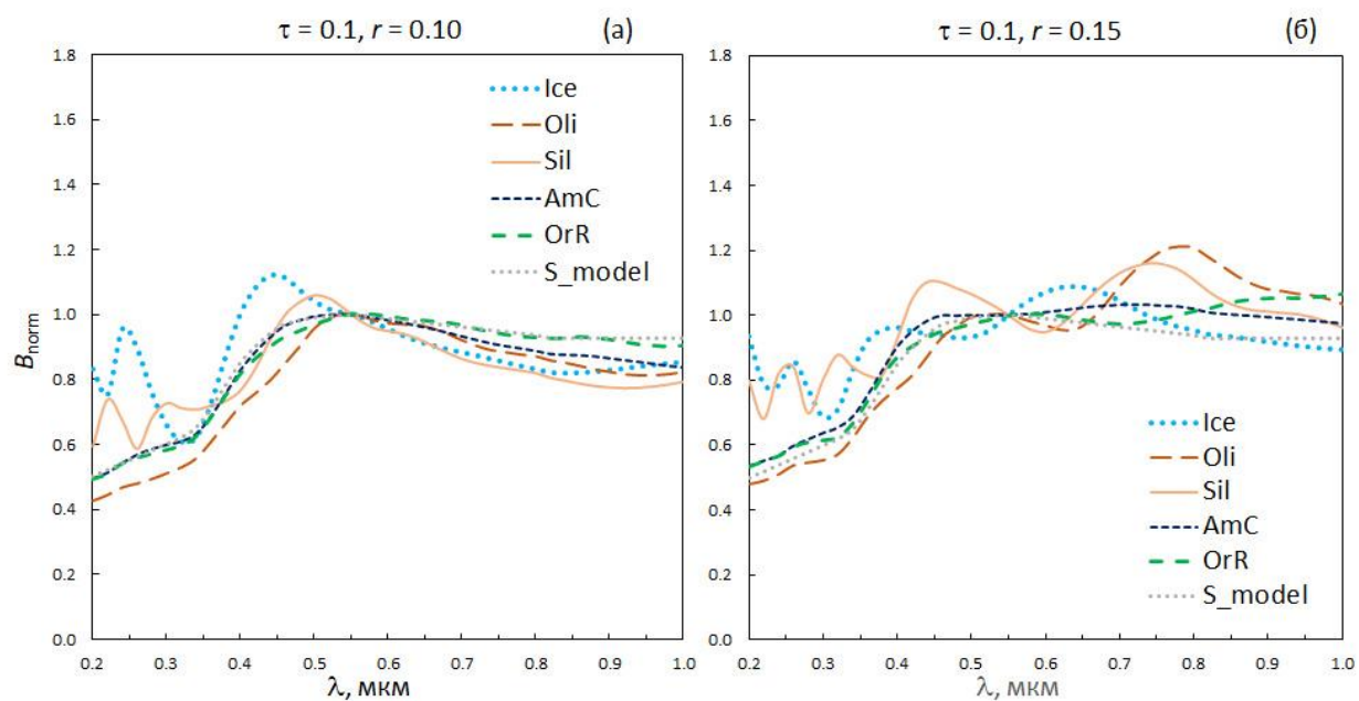
Рис. 11. То же, что на рис. 10, но для \tau = 0.1 .
