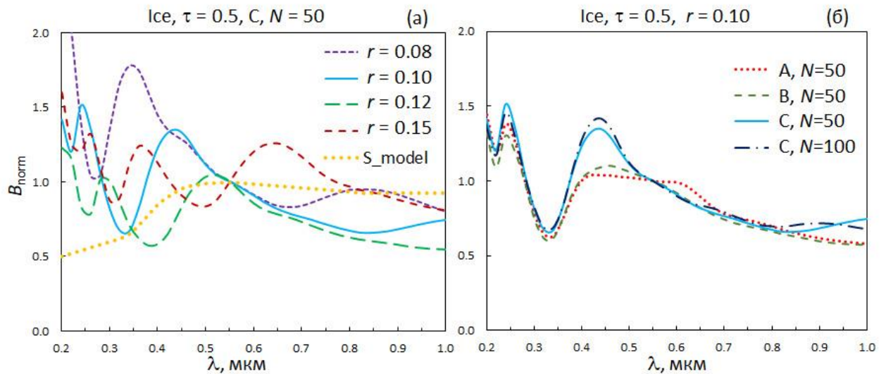
Рис. 9. Спектры B_{\text{norm}} для экзосферы оптической толщины \tau = 0.5 над поверхностью с альбедо A_s(\lambda=0.55 \text{ мкм}) = 0.072 и его нормированной спектральной зависимостью, показанной кривой S_{\text{model}} . Экзосфера состоит из ледяных агрегатов структуры C , содержащих 50 мономеров указанных радиусов r (а), и разных структур при r = 0.10 мкм и N = 50 и 100 (б).
