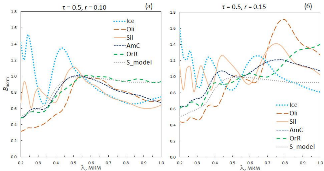
Рис. 10. Спектры B_{\text{norm}} для экзосферы оптической толщины \tau = 0.5 , состоящей из агрегатных частиц разного состава. Структуры типа С содержат 50 мономеров радиусом 0.10 мкм (а) и 0.15 мкм (б).
