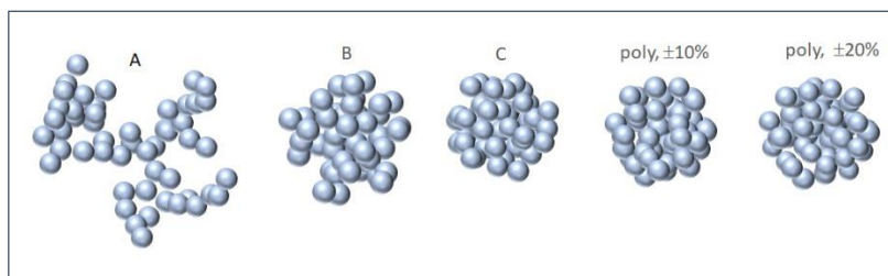
Рис. 2. Агрегатные структуры, для которых проводились расчеты характеристик рассеяния.
