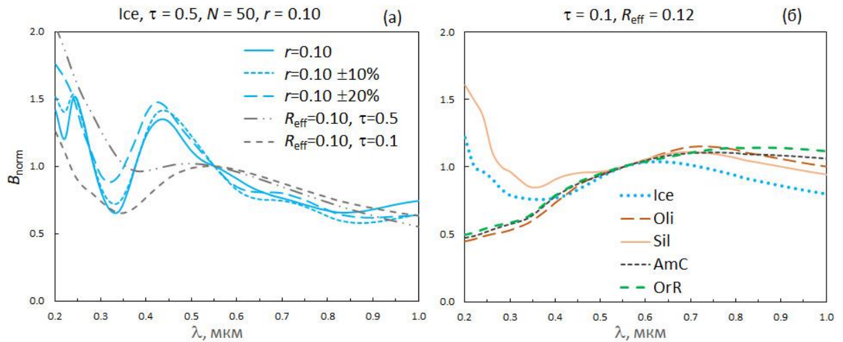
Рис. 12. (а) – Спектры B_{\text{norm}} для экзосферы, состоящей из ледяных агрегатов, радиус СЧ которых r = 0.10 мкм или варьирует в указанных пределах (при \tau = 0.5 ), или из однородных частиц при указанных размерах R_{\text{eff}} и \tau . (б) – Экзосфера с оптической толщиной \tau = 0.1 состоит из однородных частиц разного состава ( R_{\text{eff}} = 0.12 мкм).
