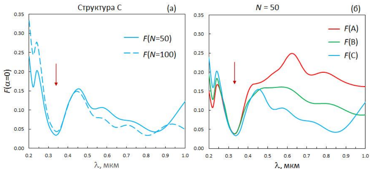
Рис. 6. Спектральные зависимости F(\alpha=0^\circ) для агрегатных ледяных частиц с мономерами радиусом 0.1 мкм. (а) – Модели для разного числа мономеров в агрегатах структуры С. (б) – Модели для агрегатов разных структур (А, В и С) при числе мономеров N = 50 . Положения первого минимума ( \lambda_1 ), сформированного интерференцией при рассеянии на отдельных СЧ, отмечены стрелками на этом и следующем рисунке.
